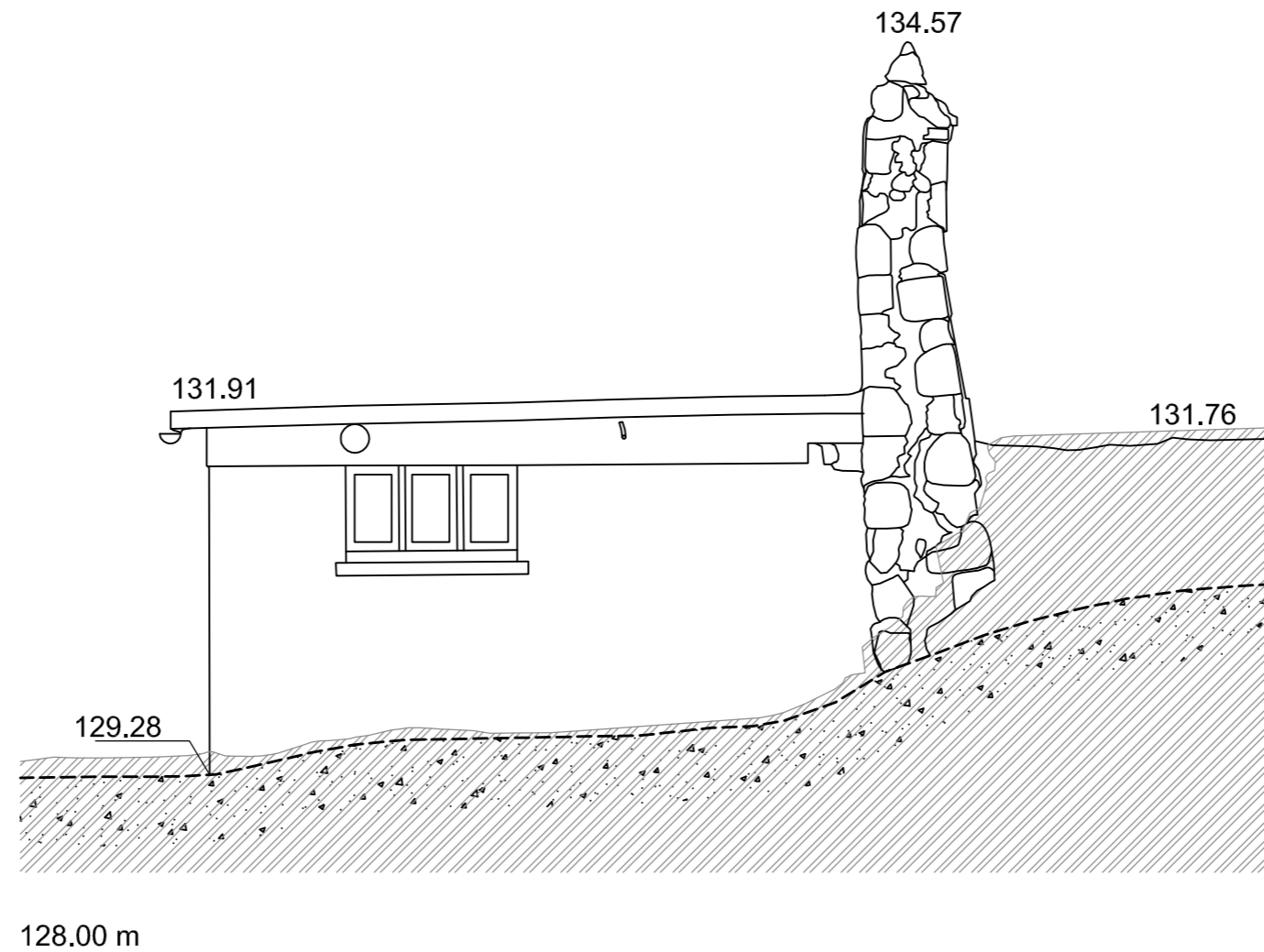
Coupe transversale C - C'
